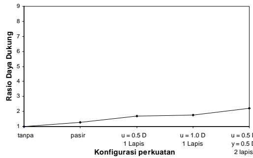
Gambar 9. Grafik hubungan rasio daya dukung dengan konfigurasi perkuatan pasir 1.0D ( D = diameter pondasi) dan anyaman bambu terletak pada lapisan pasir
